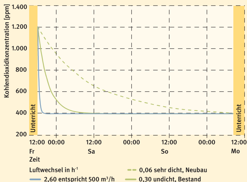
Abb. 12 Abnahme der CO 2 -Konzentration in einem Klassenzimmer bei unterschiedlichen Luftwechseln nach Unterrichtsschluss an einem Freitag um 15:00 Uhr, Ausgangskonzentrationen CO 2 innen: 1.200 ppm, außen: 400 ppm Quelle: Hellwig
