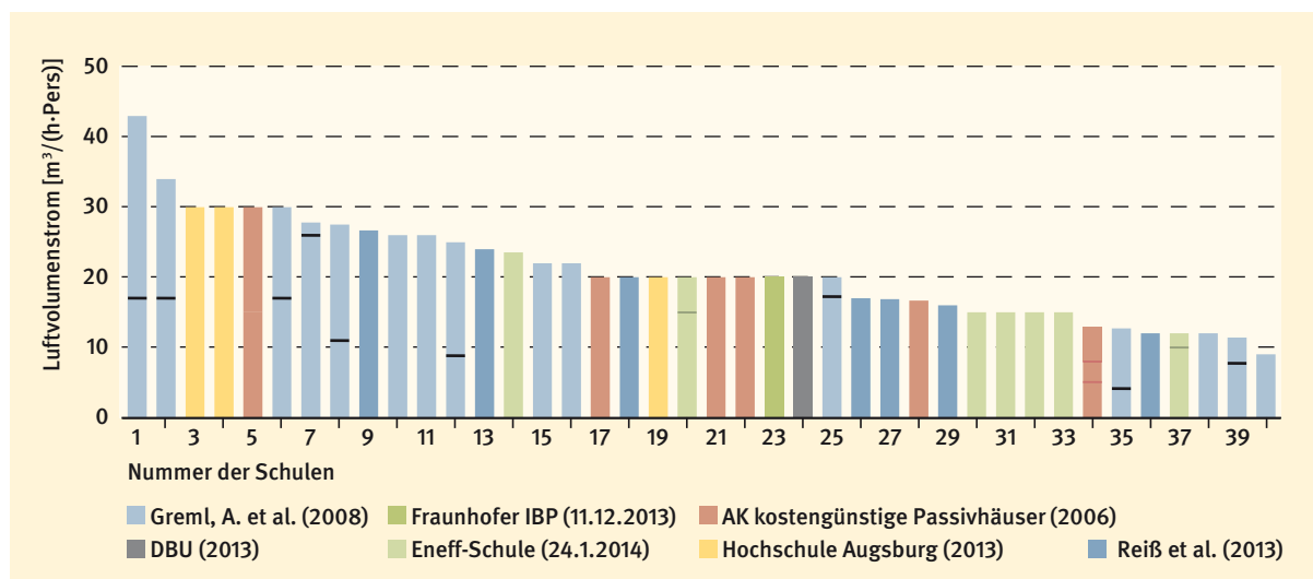
Abb. 7 In Demonstrations- und Praxisprojekten in Deutschland und Österreich umgesetzte Luftmengen bei Gebäuden mit mechanischen Lüftungsanlagen Quelle: Hackl, Hellwig
