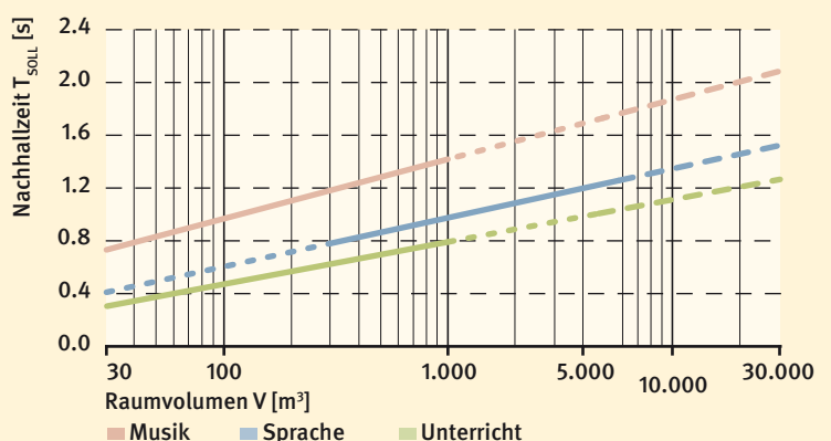
Abb. 18 Werte für die Nachhallzeit T_{soll} je nach Raumnutzung und -volumen nach DIN 18041 Quelle: Akustikbüro Oldenburg
